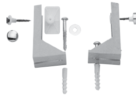
733 € 2,40 Coppia zanche in plastica antiurto a L con viti, per fissaggio laterale W.C. e bidet. Couple wall brackets in plastic, shock-resistant, L shaped, with screws, for side WC and bidet fixing.
